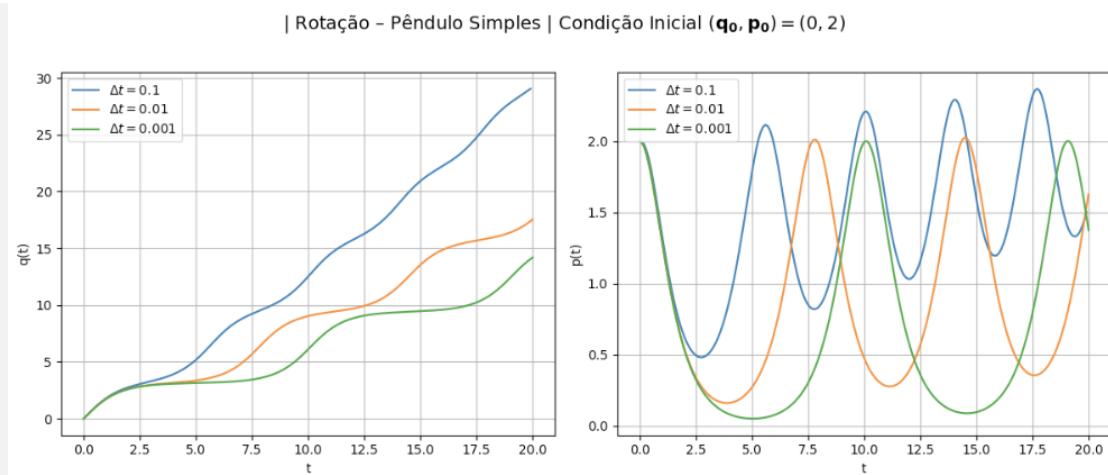
Figure 2: Evolução temporal do momento canônico p(t) usando o Método de Euler Convencional.
